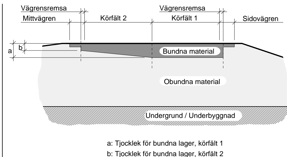
Figur 4.4-1 Trapetsformad tjockleksförändring
