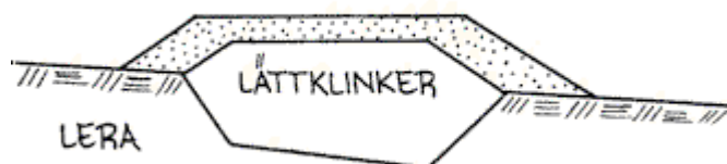
Fig 1.2 Kompensationsgrundläggning
